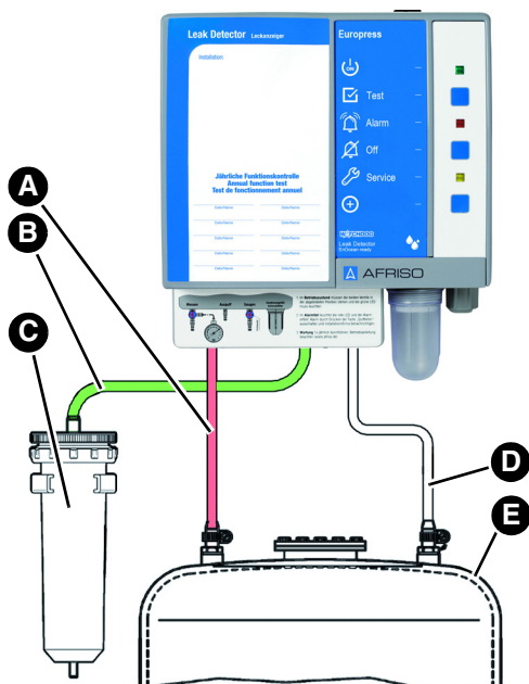
Abbildung 2: Aansluiten van een bovengrondse tank
