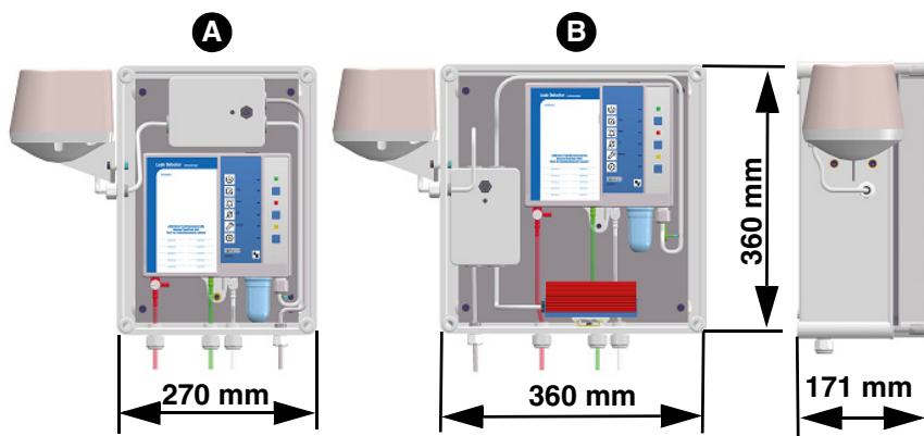
Figura 1: Europress in involucro protettivo, senza (A) oppure con (B) riscaldamento, preassemblato per la connessione. L'avvisatore acustico è collegato al relè d'uscita. Grado di protezione IP 55.
